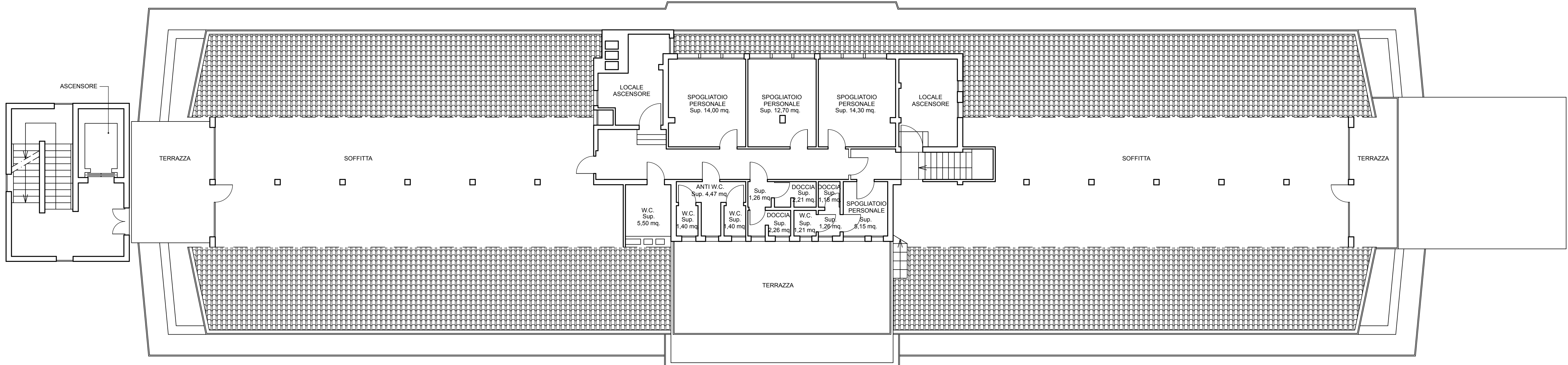
PIANTA PIANO SETTIMO AREA SERVIZI
