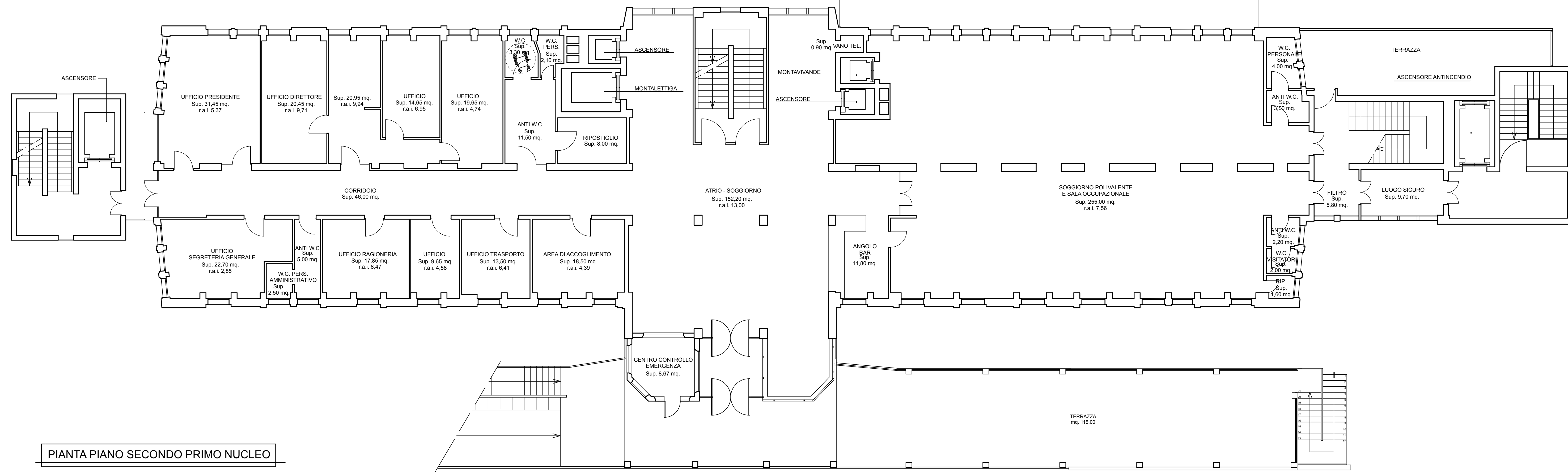
PIANTA PIANO PRIMO AREA SERVIZI - C.D.I.
